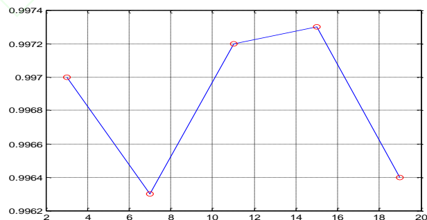
图 9 卷积核大小与分类性能的影响
